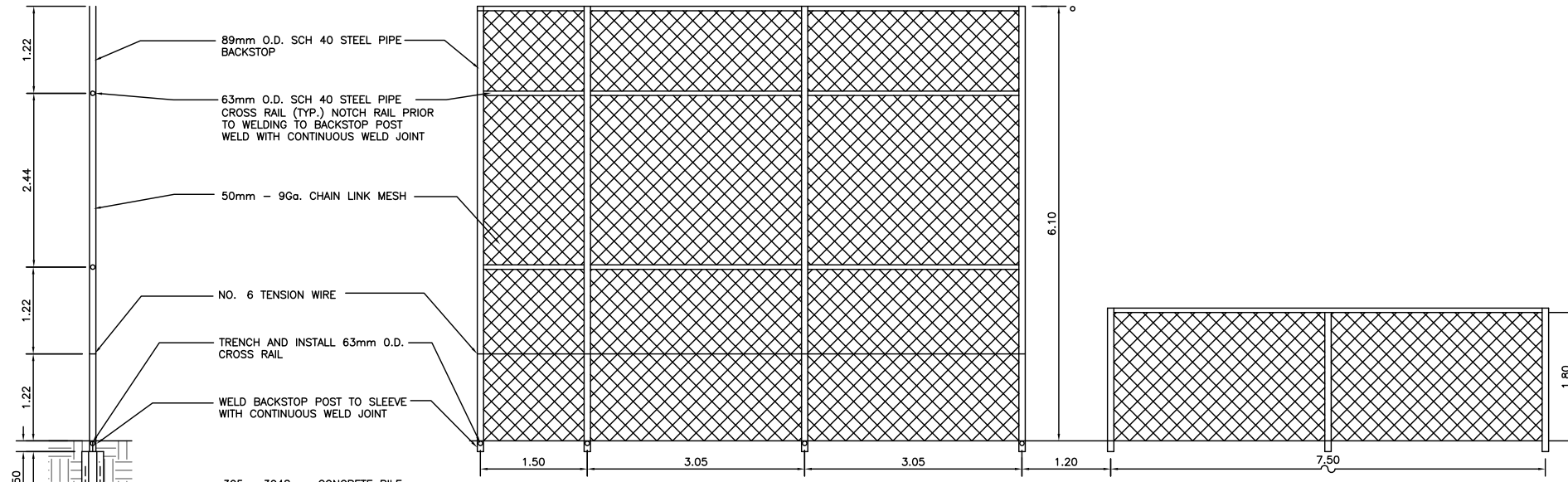
ELEVATION
